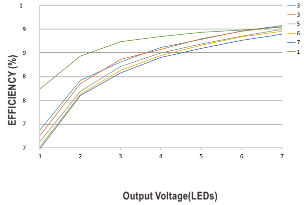
Fig-2 24VDC input, 1~7 LEDs( V_f=3V )
